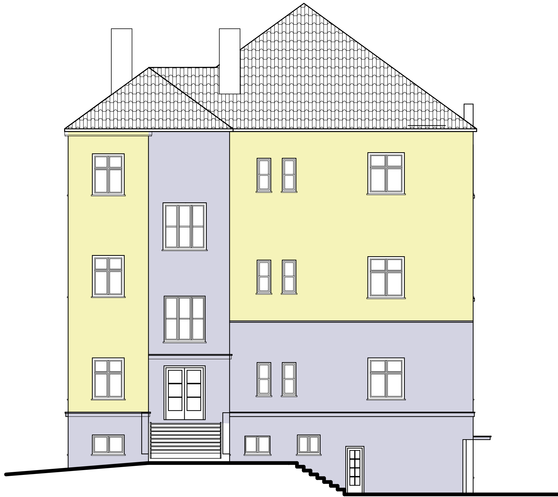
Pohled Jižní
